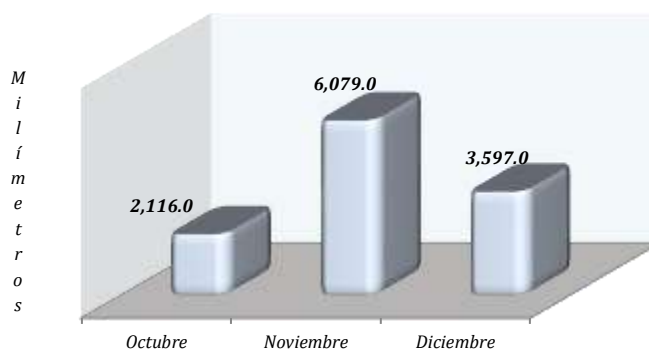
La Pampa. Acumulado de Precipitaciones - 4º Trimestre 2017
